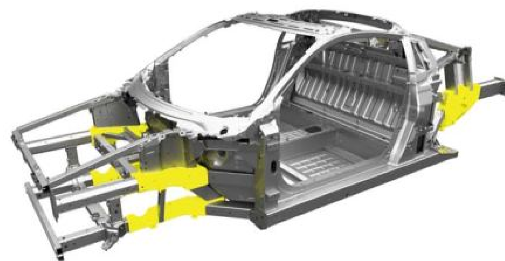
▲ NSX 全車六處的切割鑄造鋁合金車樑銲點，在結構力學上達到更輕量卻更堅固的需求。
