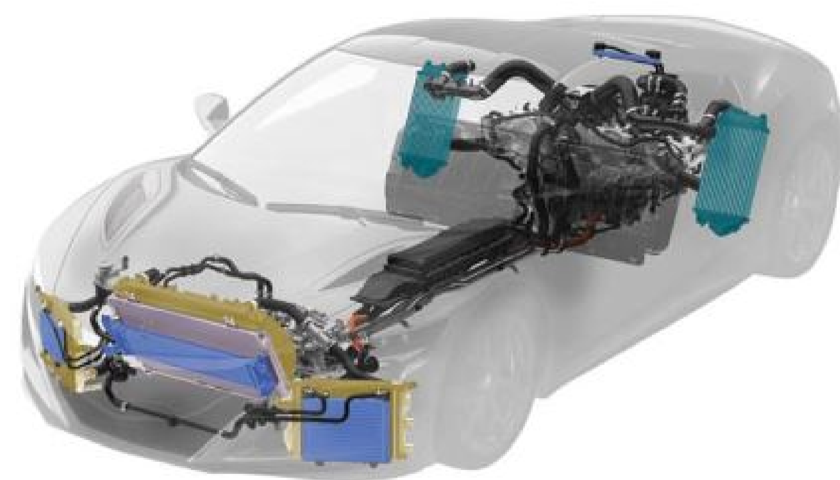
▲ NSX 內部動力系統共配備十組散熱器，讓流經車內的氣流迅速帶走運轉時產生的高熱。
