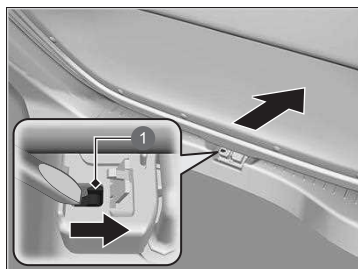
① 鎖扣桿
